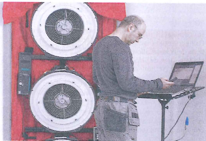
Un test d'infiltrométrie réalisé par le réseau Rhizome. © D. DEVROEY.
